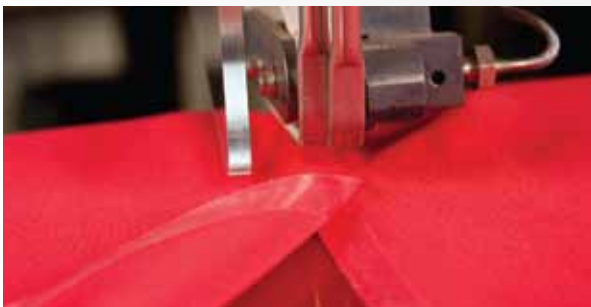
União de Materiais por calor. 2 sopradores superiores, além de aquecimento das correias superior e inferior.
